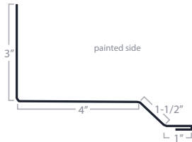
Sidwall
