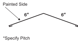
Hip Cap
