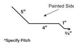
Endwall
