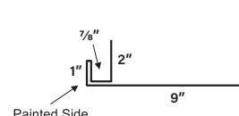
Overhead Door Jamb
