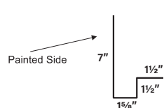
DJ8 Jamb Trim
