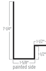
DJ8 JAMB TRIM
