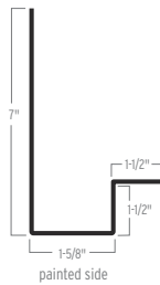
DJ8 JAMB TRIM
