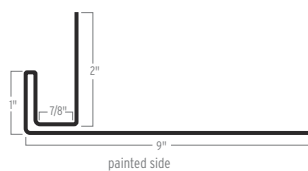
OVERHEAD DOOR JAMB
