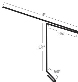
D-EDGE
