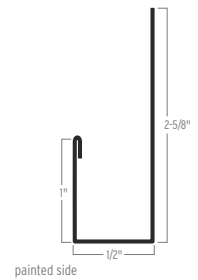
SOFFIT J-TRIM
