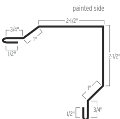
MINI CORNER/RAKE
