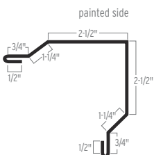
MINI CORNER/RAKE
