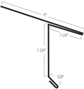
D-EDGE
