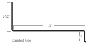
SOFFIT BOX
