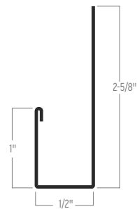
SOFFIT J-TRIM
